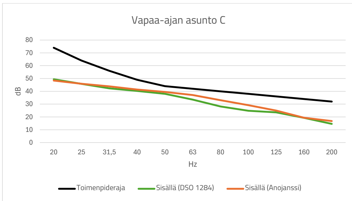
Kuva 6. Ympäristöministeriön ohjeistuksen mukainen pienitaajuisen melun laskenta sekä sosiaali- ja terveysministeriön toimenpiderajat vapaa-ajan asunnossa C.
