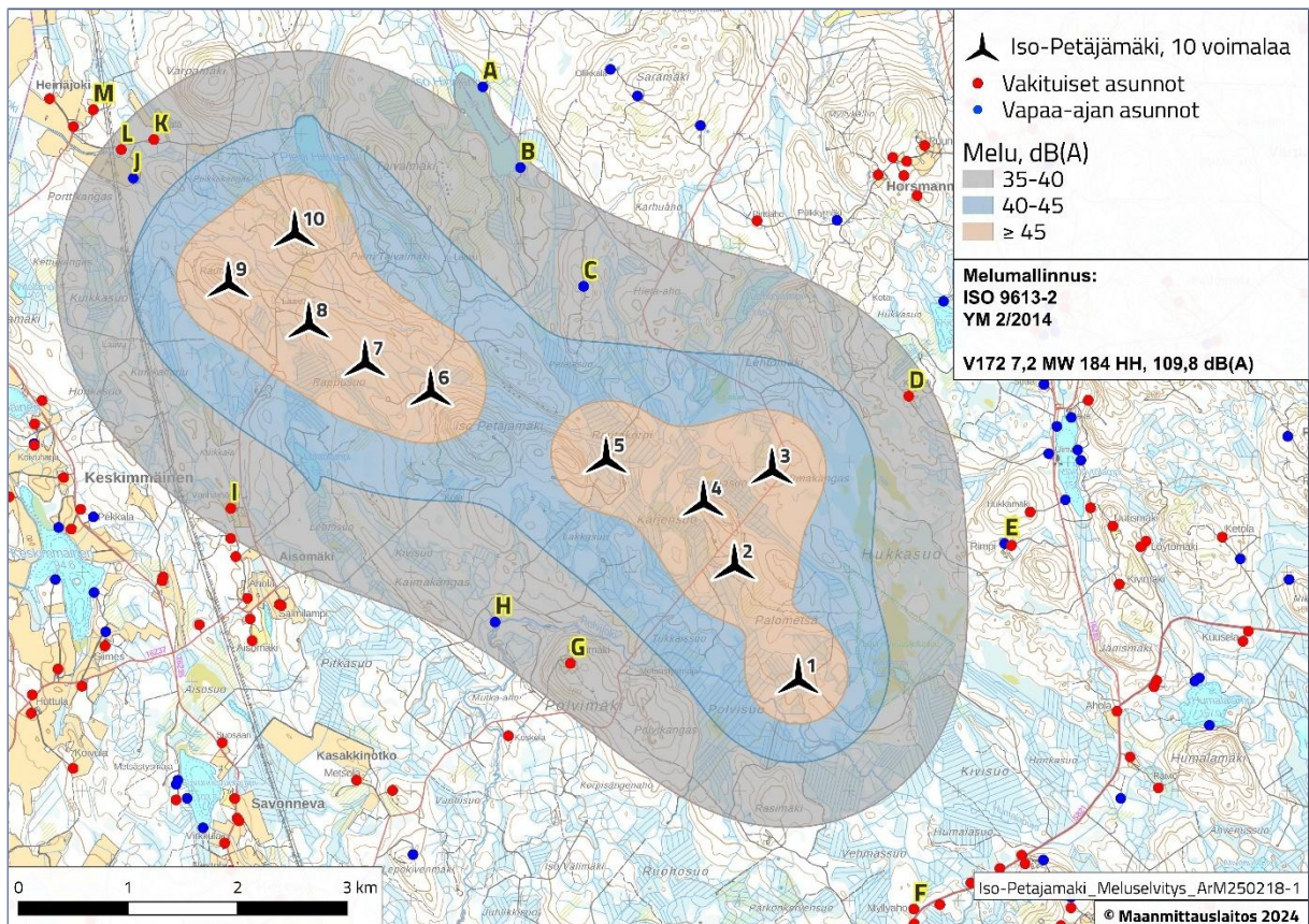
Kuva 1. Iso-Petäjämäen tuulivoimapuiston melumallinnus, V172 7,2 MW 184 HH, 107,8 +2 dB(A). 13 havainnointipistettä on merkitty kuvaan kirjaimilla.
