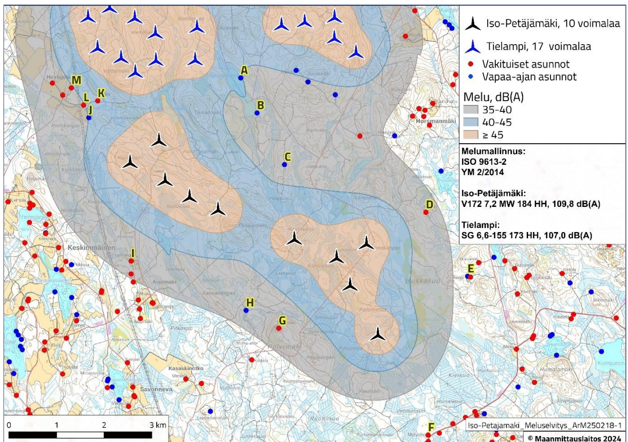
Kuva 2. Iso-Petäjämäen (10 voimalaa) ja naapuripuiston yhteisvaikutusten melumallinnus.
