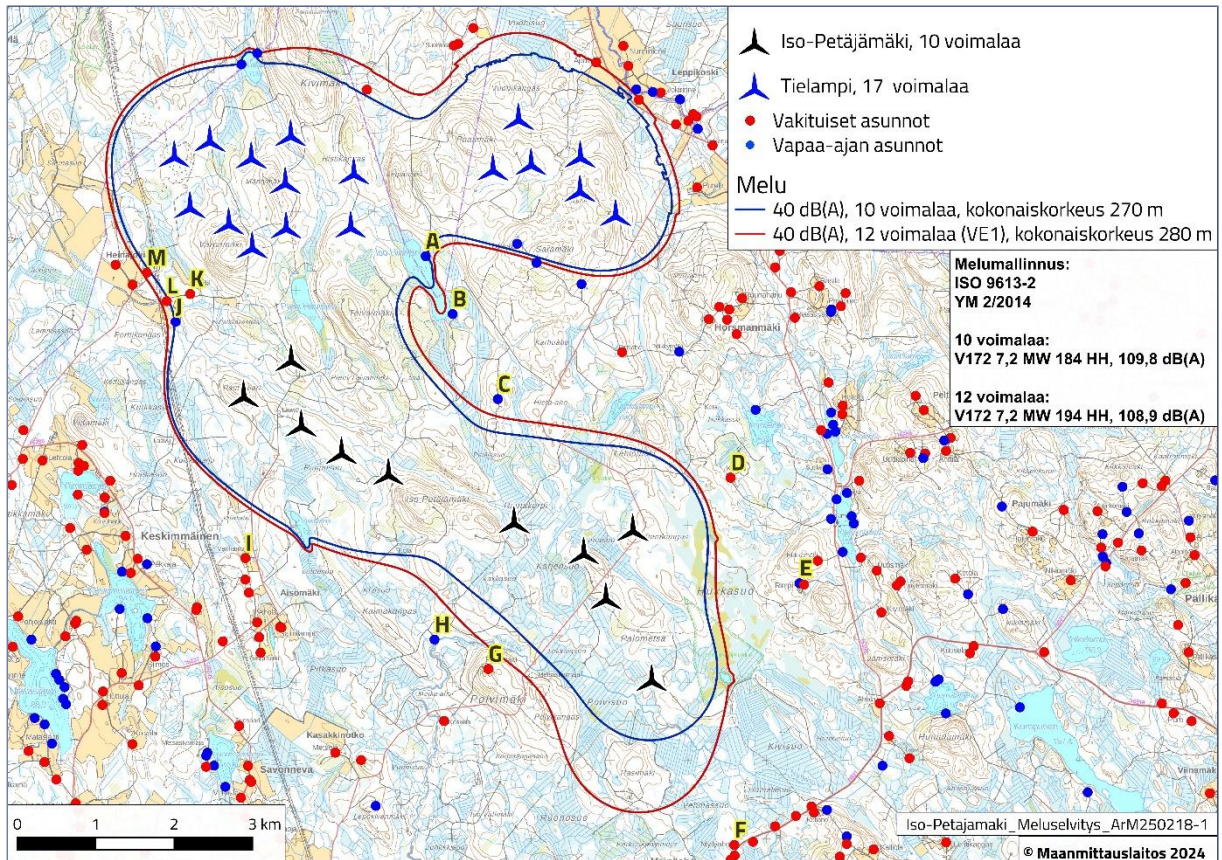
Kuva 8. Iso-Petäjämäen (10 voimalaa) ja naapuripuiston yhteisvaikutusten melumallinnus. Kuvassa on esitetty rajat, joiden sisäpuolella ylitetään valtioneuvoston asetuksen ohjearvo 40 dB(A).
