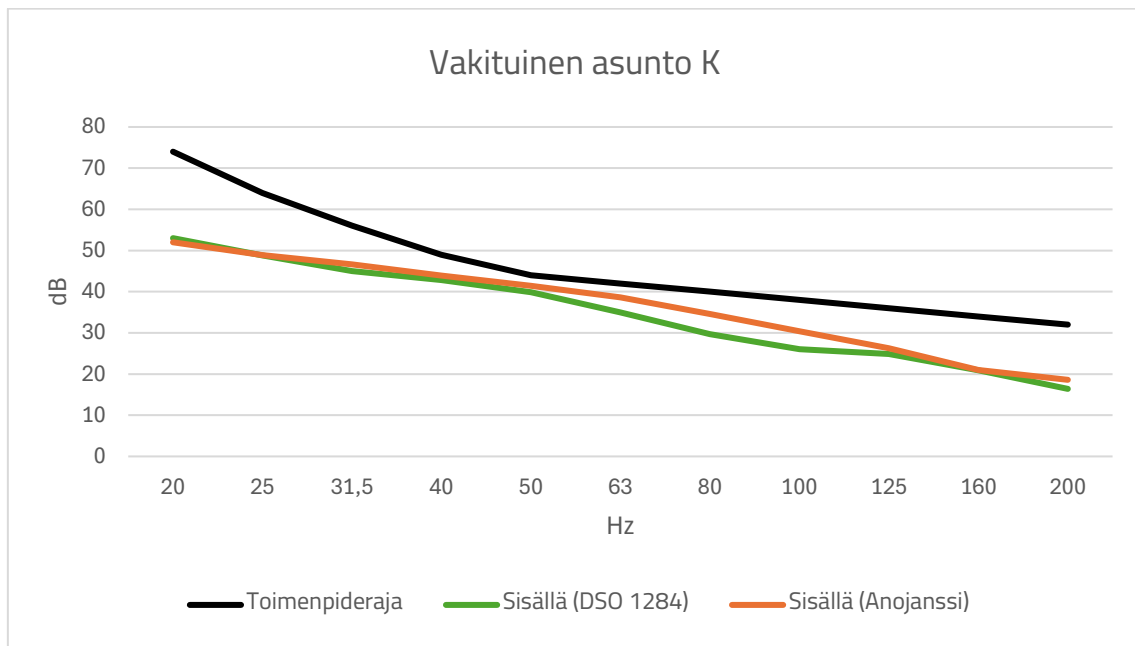
Kuva 5. Ympäristöministeriön ohjeistuksen mukainen pienitaajuisen melun laskenta sekä sosiaali- ja terveysministeriön toimenpiderajat vakituksessa asunnossa K.
