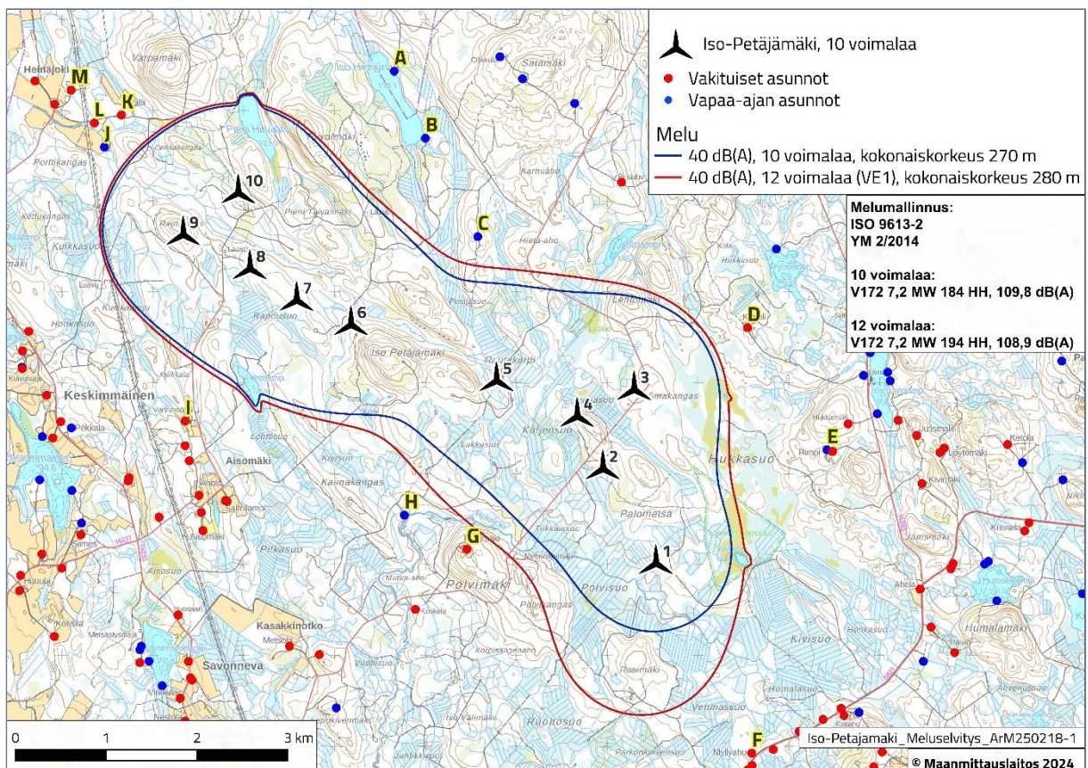
Kuva 7. Iso-Petäjämäen tuulivoimapaiston melumallinnus. Kuvassa on esitetty rajat, joiden sisäpuolella ylitetään valtioneuvoston asetuksen ohjearvo 40 dB(A).
