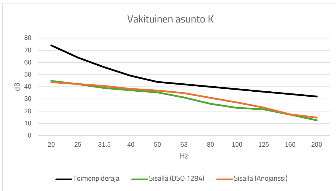
Kuva 3. Ympäristöministeriön ohjeistuksen mukainen pienitaajuisen melun laskenta sekä sosiaali- ja terveysministeriön toimenpiderajat vakituksessa asunnossa K.
