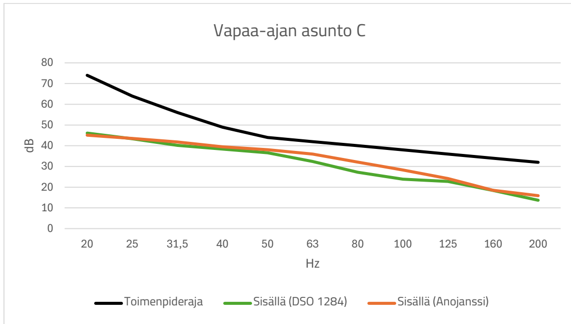
Kuva 4. Ympäristöministeriön ohjeistuksen mukainen pienitaajuisen melun laskenta sekä sosiaali- ja terveysministeriön toimenpiderajat vapaa-ajan asunnossa C.
